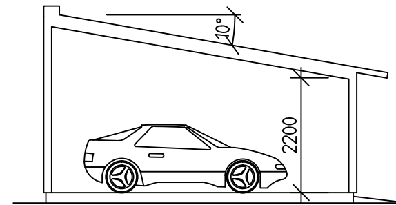
FASAD VÄSTER
